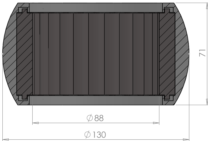
SECTION A-A SCALE 1 : 1.25
